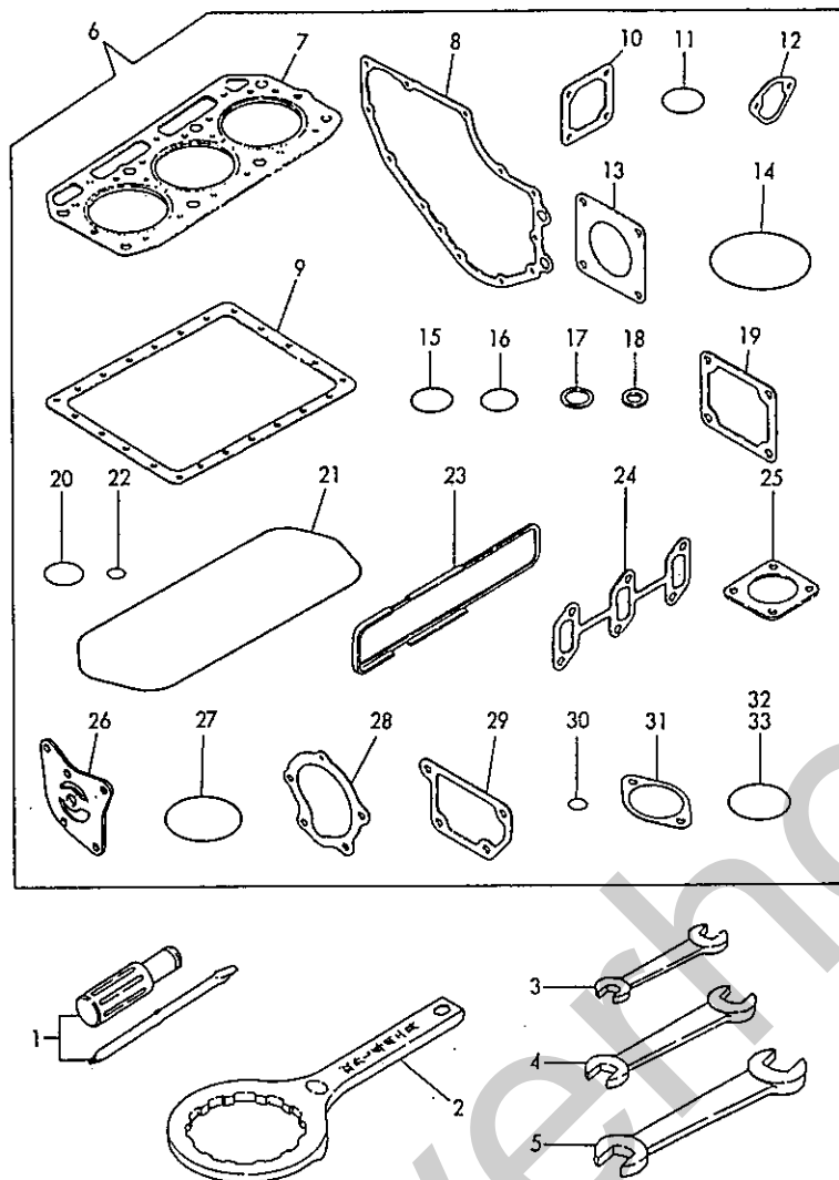
Fig. 40 パッキンセット(オプション)&コウグ GASKET SET (OPTIONAL) & TOOL
