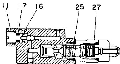
SECTION "A-A" 断面 "A-A"
